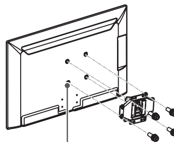
Inneres Distanzstück für Wandhalterung
