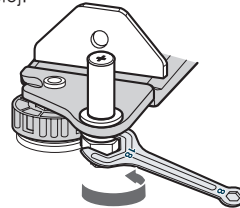
Apriete la tuerca
