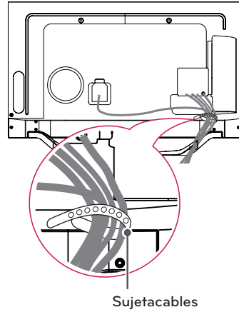
Sujetacables
