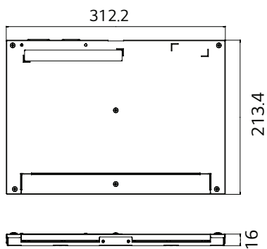
T-con Box
