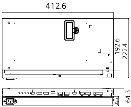
Signage Box
