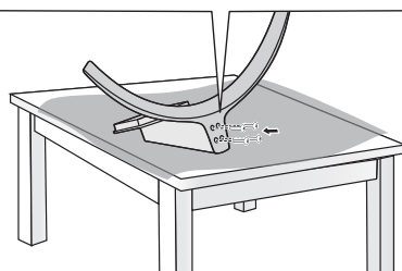
スタンド固定用ネジ (4本) M5 (長さ 25 mm)
