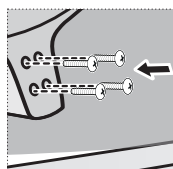
スタンド固定用ネジ (4本) M5 (長さ 25 mm)
