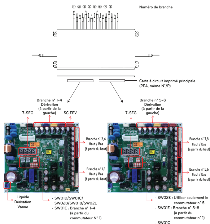
Carte à circuit imprimé principale (Maître) Carte à circuit imprimé principale (Esclave)
