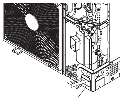
Ejecteur de tuyau pour les tuyaux de gaz/de liquide
